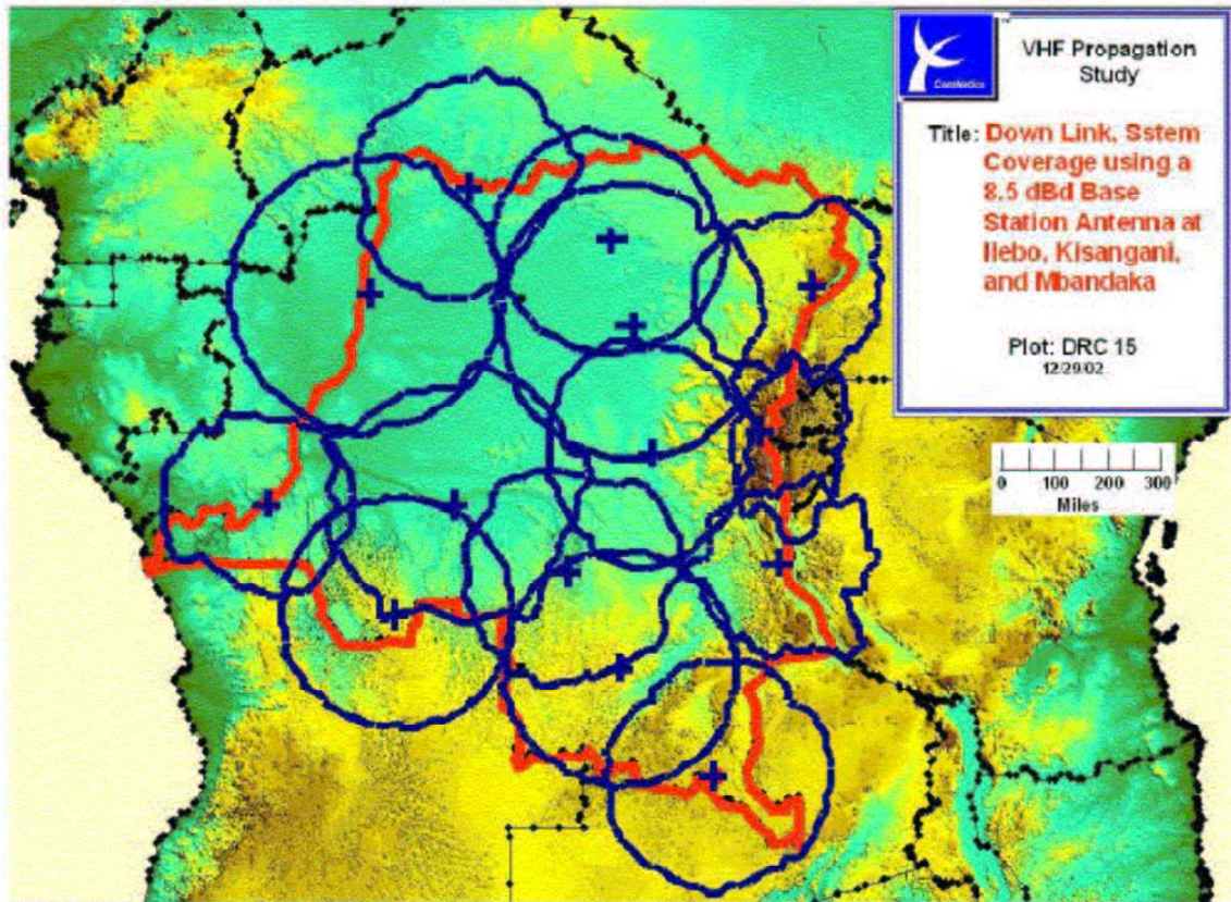
Carte des Réseaux VSAT et VHF de la RVA
