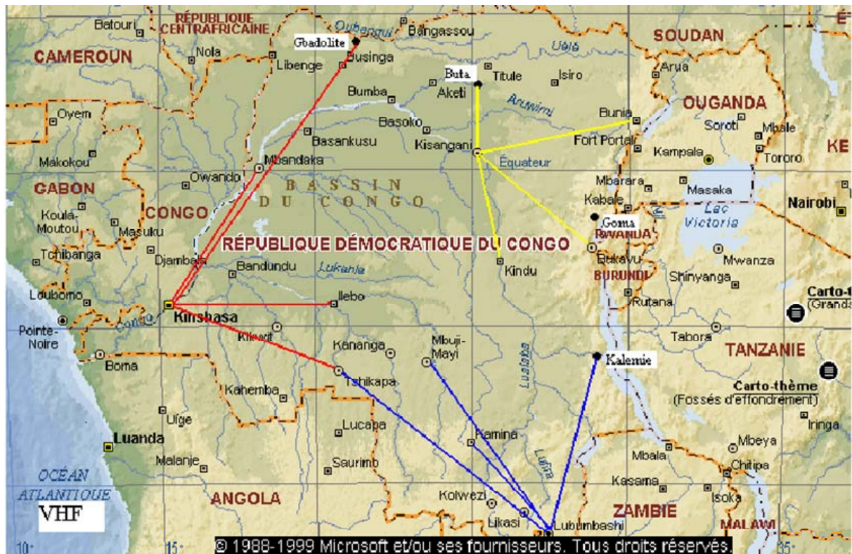
Plan d'exploitation des réseaux VHF par les trois CCR Kinshasa, Lubumbashi et Kisangani
